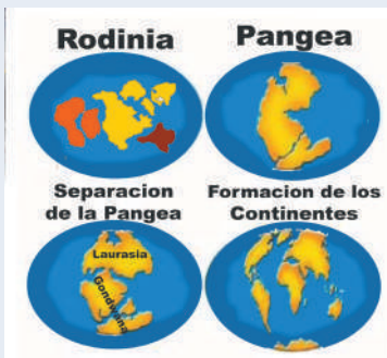
Imagen de la teoría de la derivación continental
